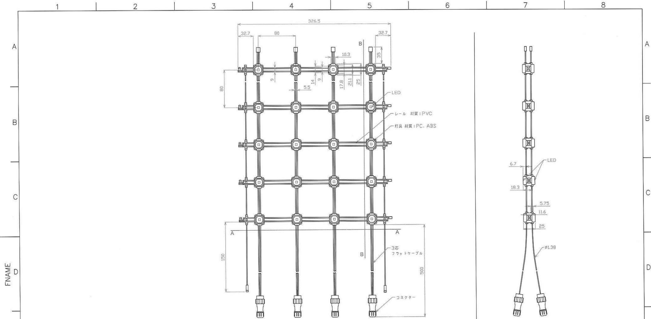
製品取付図(ネット両面)
